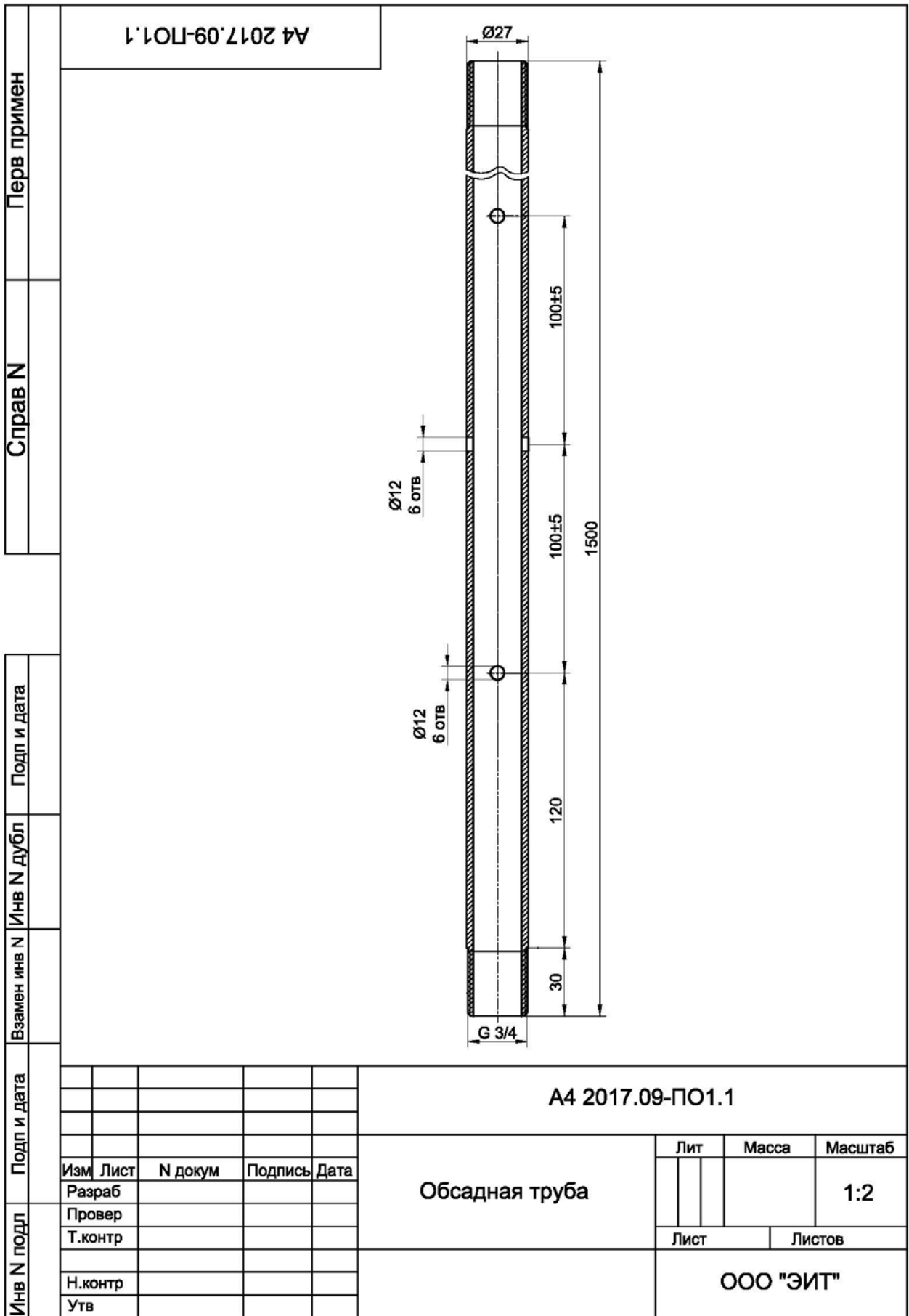
Рис.6 Обсадная труба
