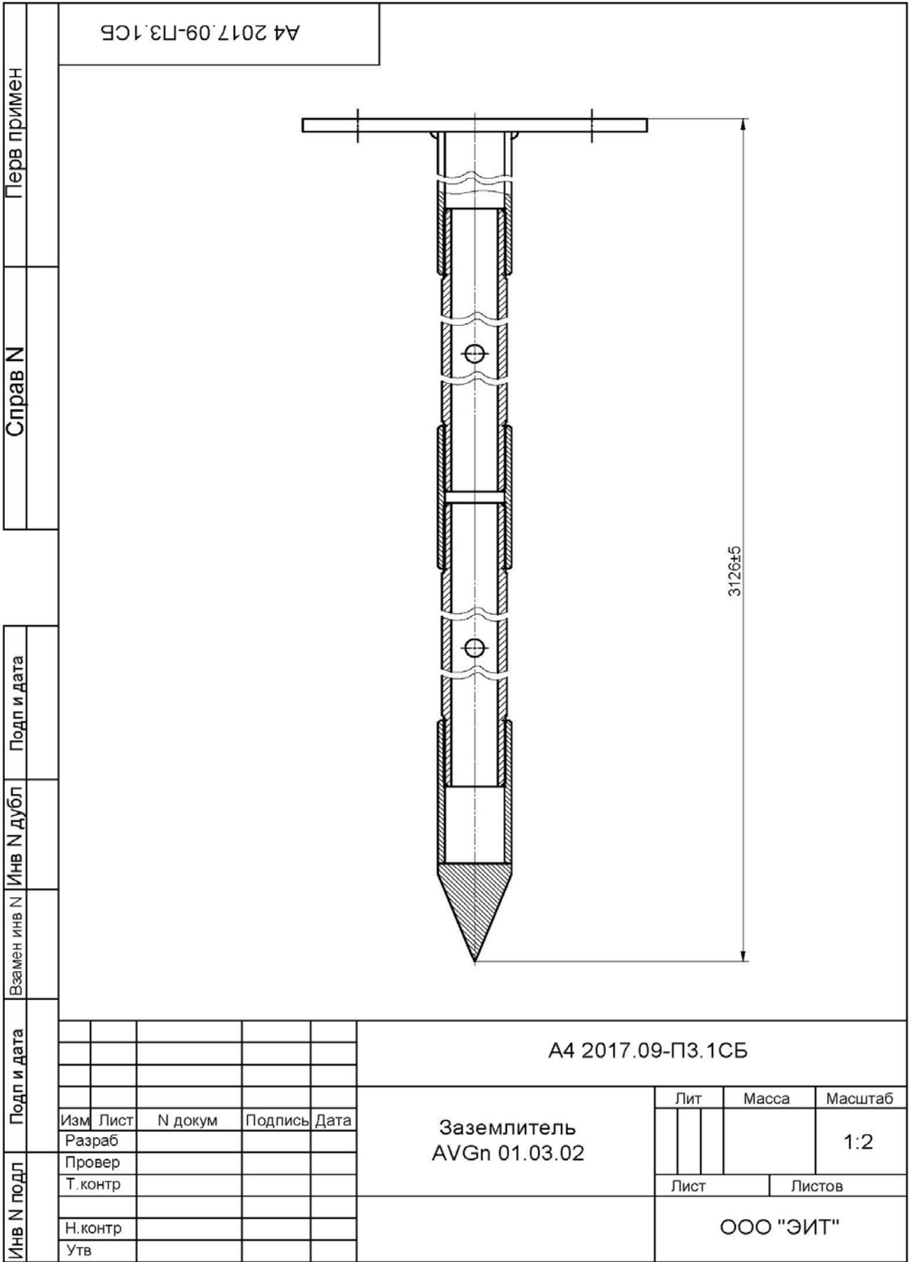
Рис.17 Заземлитель AVGn 01.03.02
